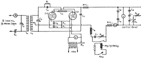
FIG. 1.—THE H.C. HARTLEY TRANSMITTER
